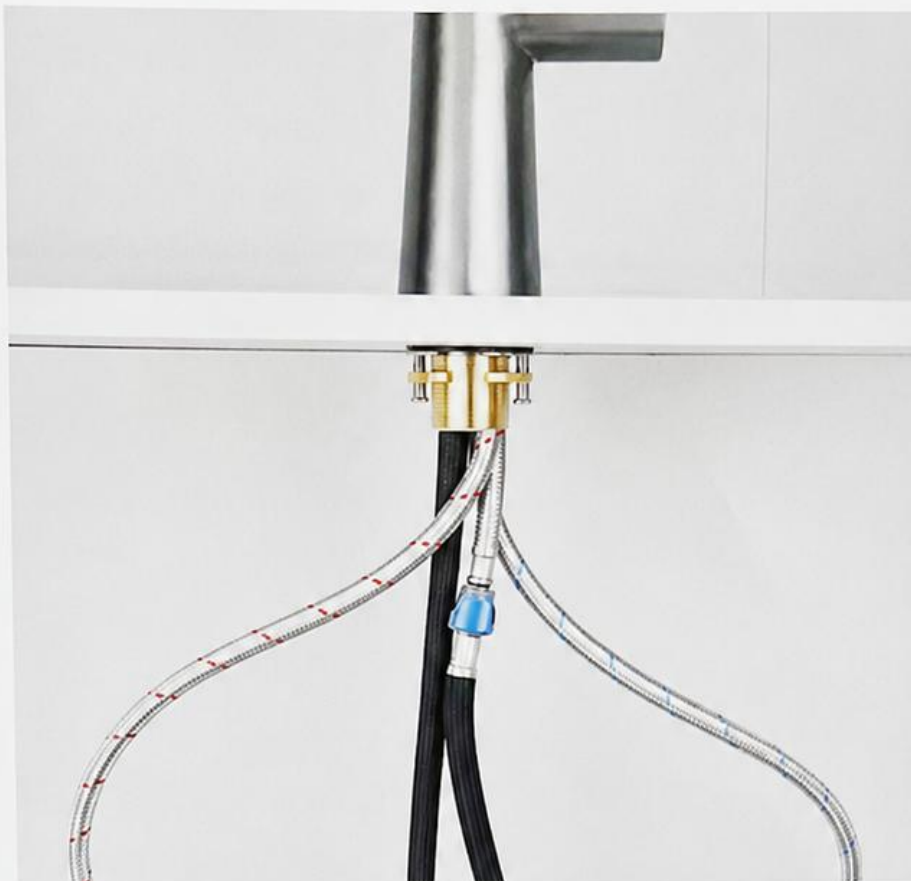
Sơ đồ hoàn tất lắp đặt
