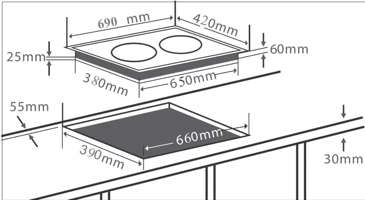
Kích thước khoét lỗ: EH-xxx2000A.
