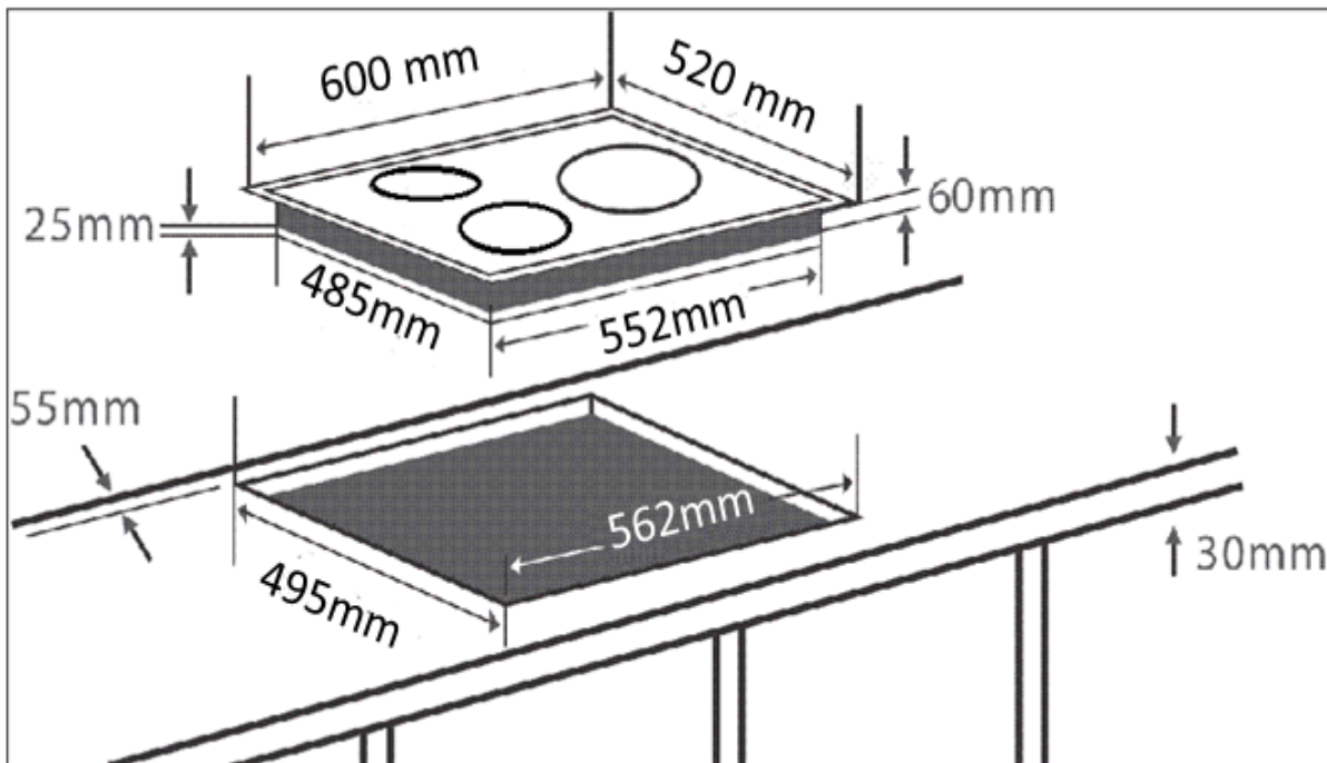
Kích thước khoét lỗ đá
