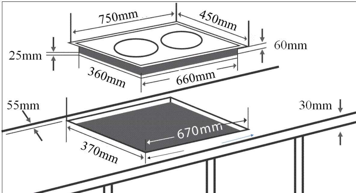
Kích thước khoét lỗ EH-DIH896.
