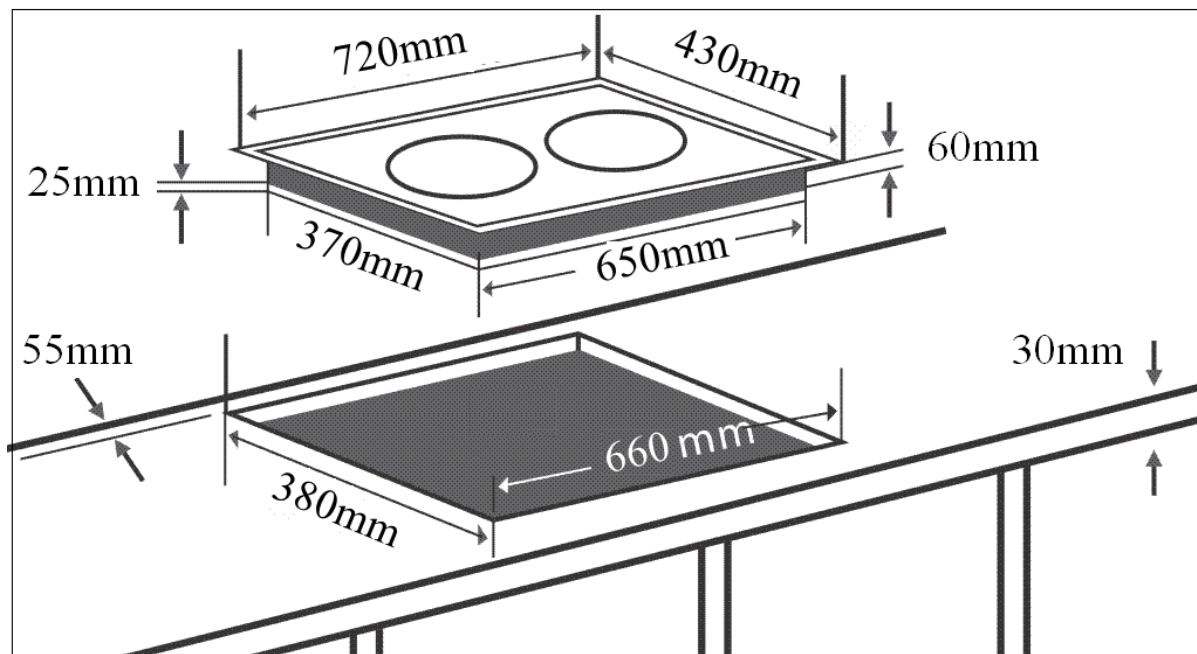
Kích thước khoét lỗ: EH-DIH989 Premium
