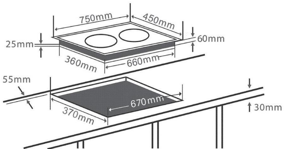
Kích thước khoét lỗ đá
