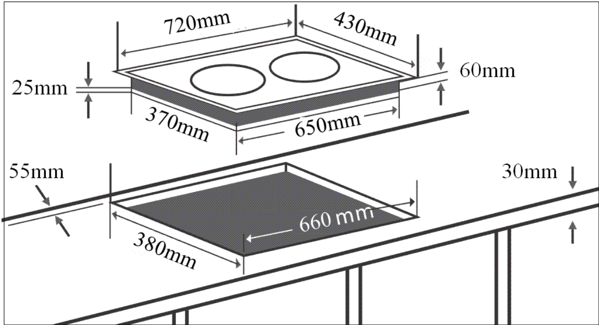
Kích thước khoét lỗ: EH – DIH320 PRO.
