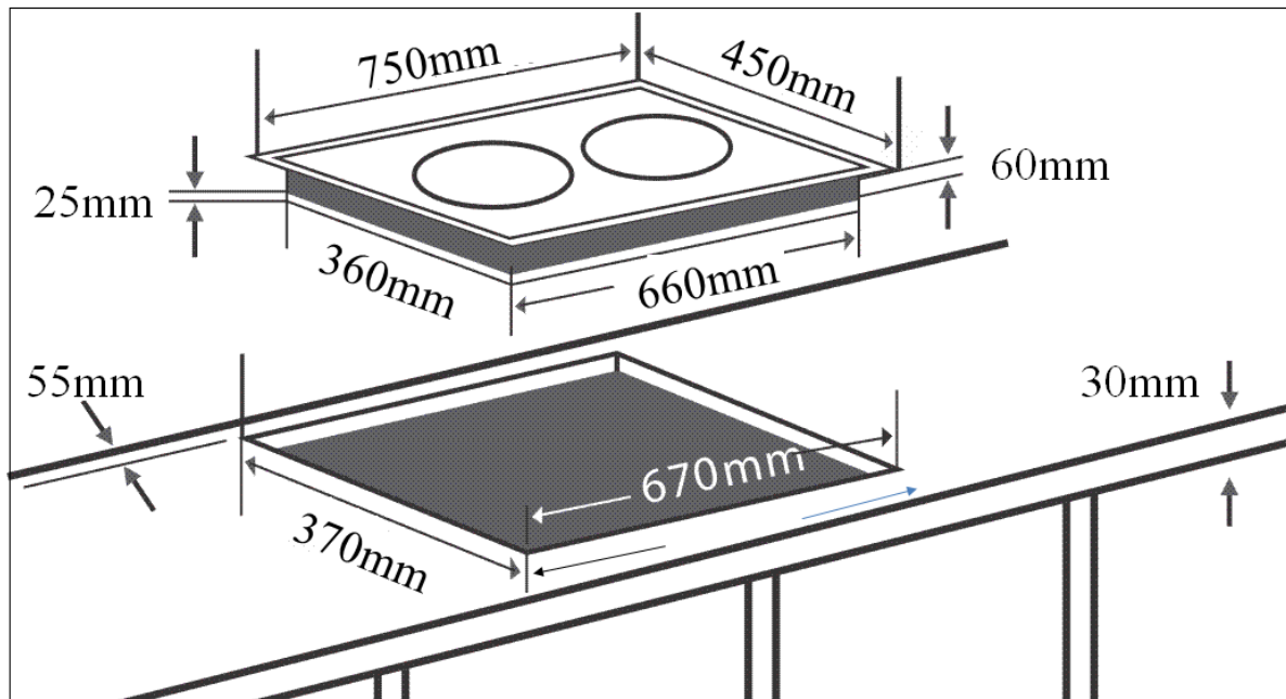
Kích thước khoét lỗ EH-DIH888 PLUS.
