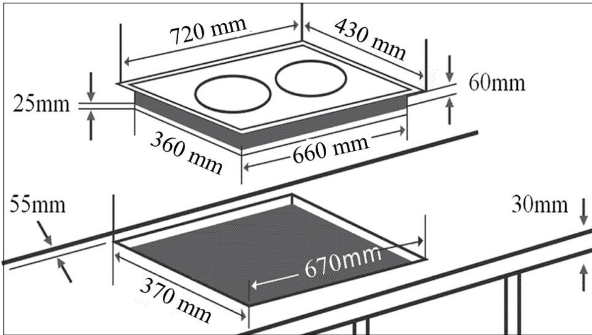
Kích thước khoét lỗ: EH-DIH389 PRO
