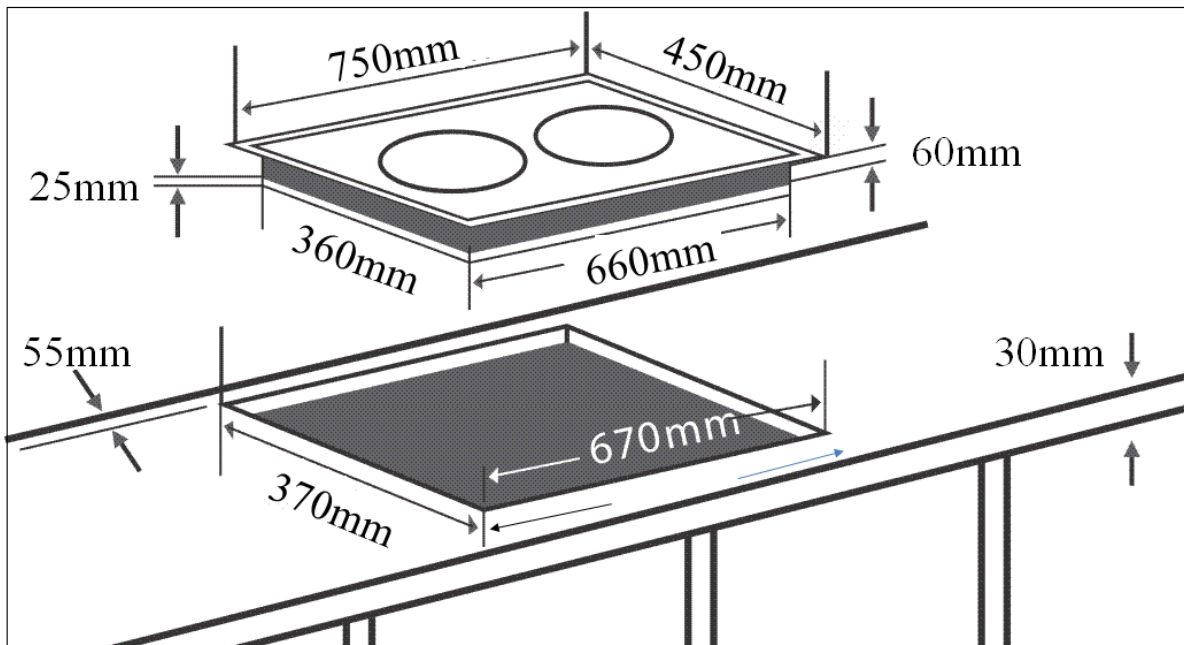
Kích thước khoét lỗ EH-DIH888 PRO.
