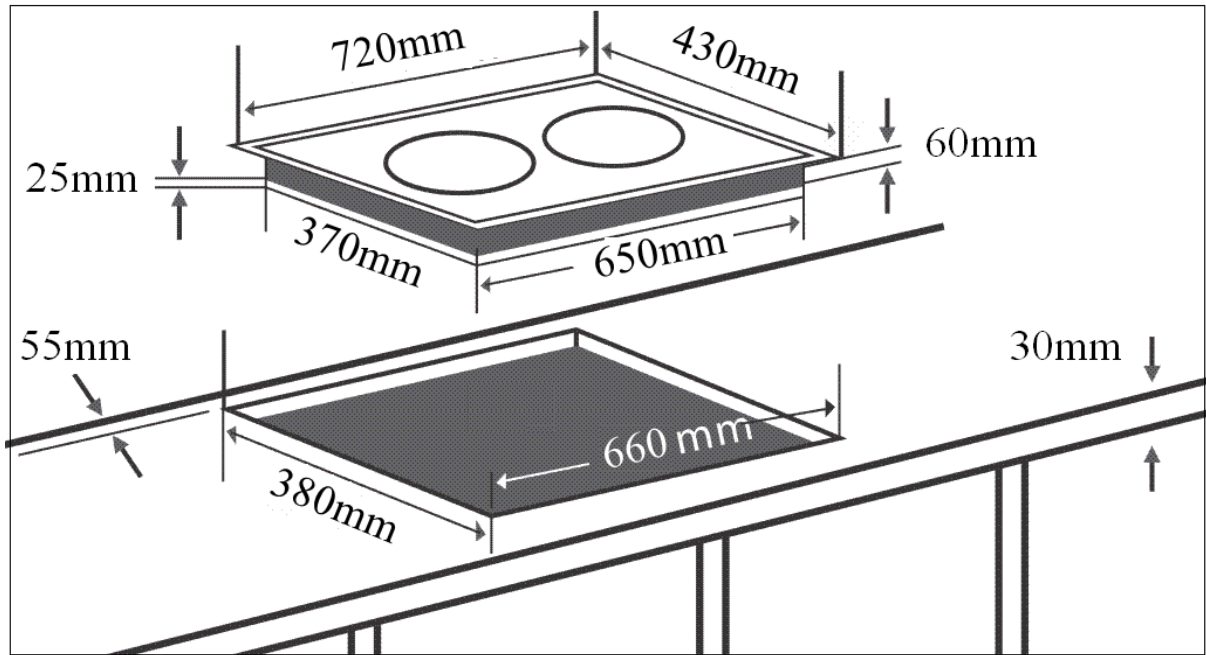
Kích thước khoét lỗ: EH – DIH300
